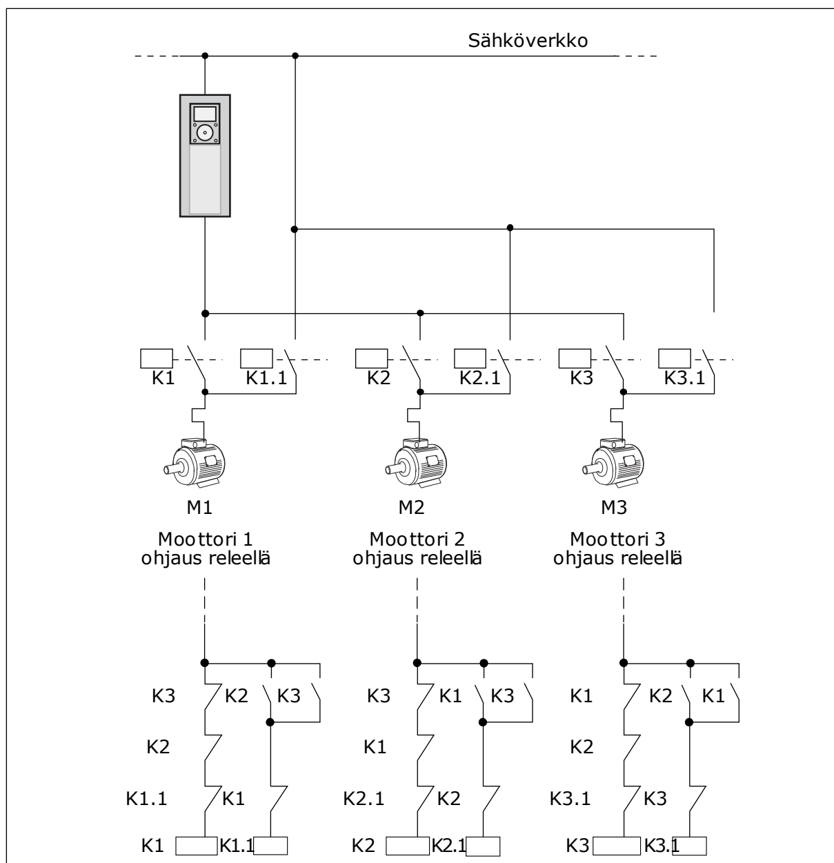
Kuva 84: Valinta 1
