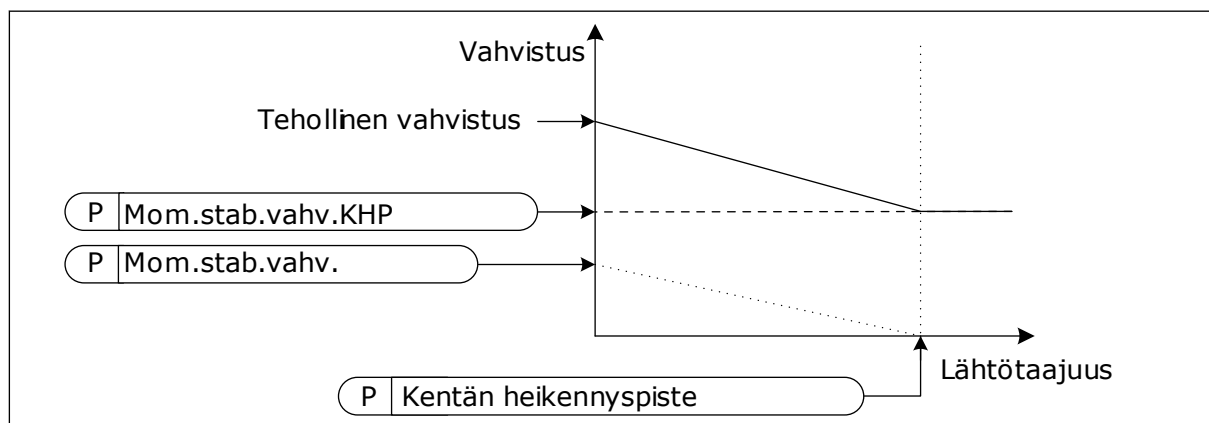
Kuva 26: Momenttistabilaattorin vahvistus
