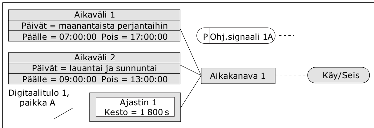
Kuva 68: Käynnistyskomennon ohjaussignaalina käytetään aikakanavaa 1 digitaalitulon sijasta.
