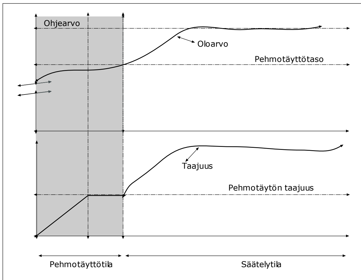
Kuva 76: Pehmotäyttötoiminto
