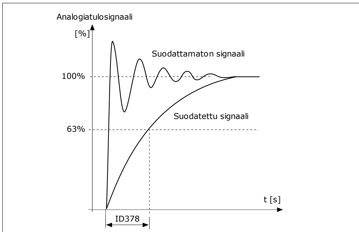
Kuva 46: AI1-signaalin suodatus.
