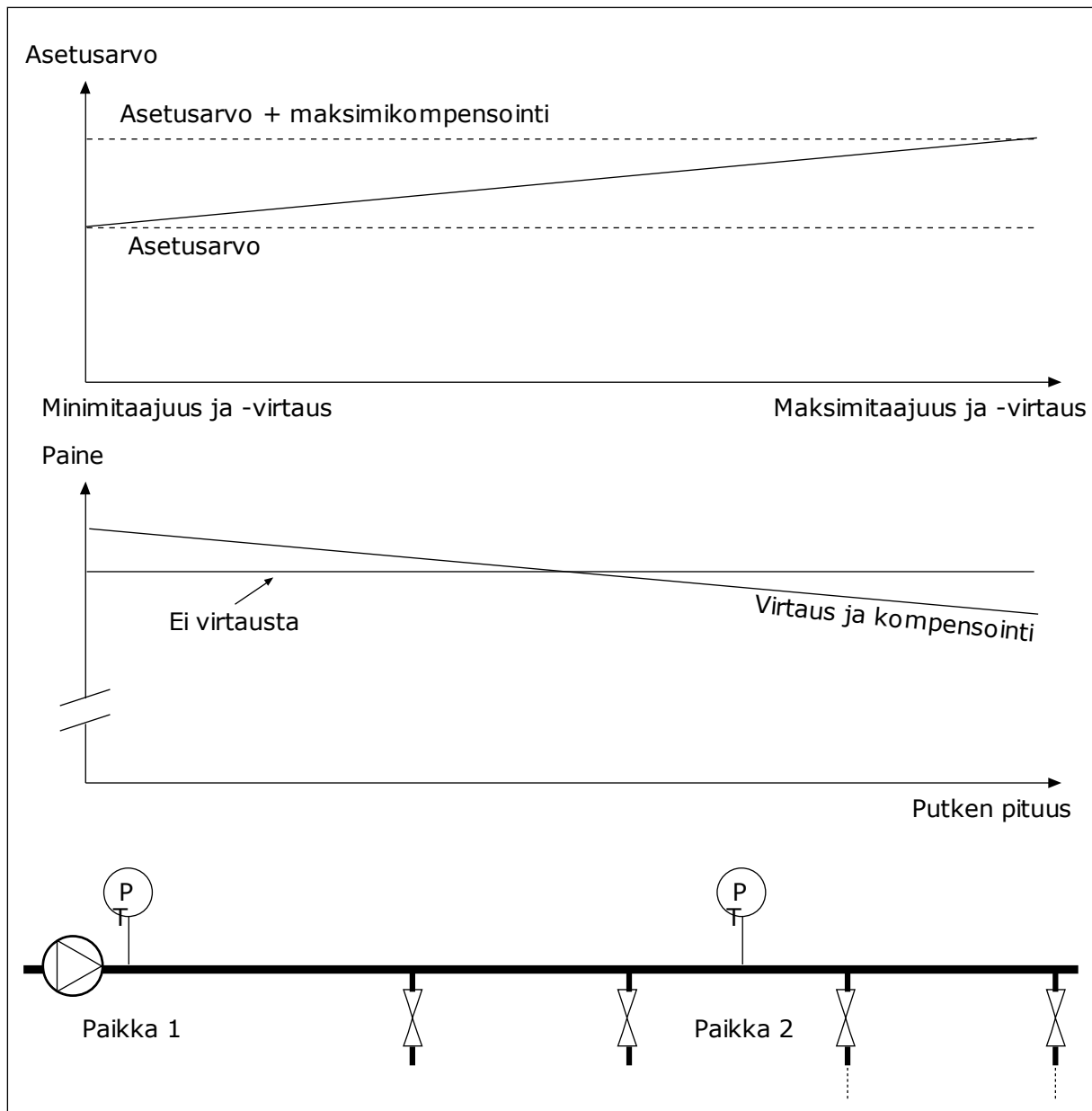
Kuva 75: Painehäviön kompensoinnin asetusarvo 1 on käytössä.
