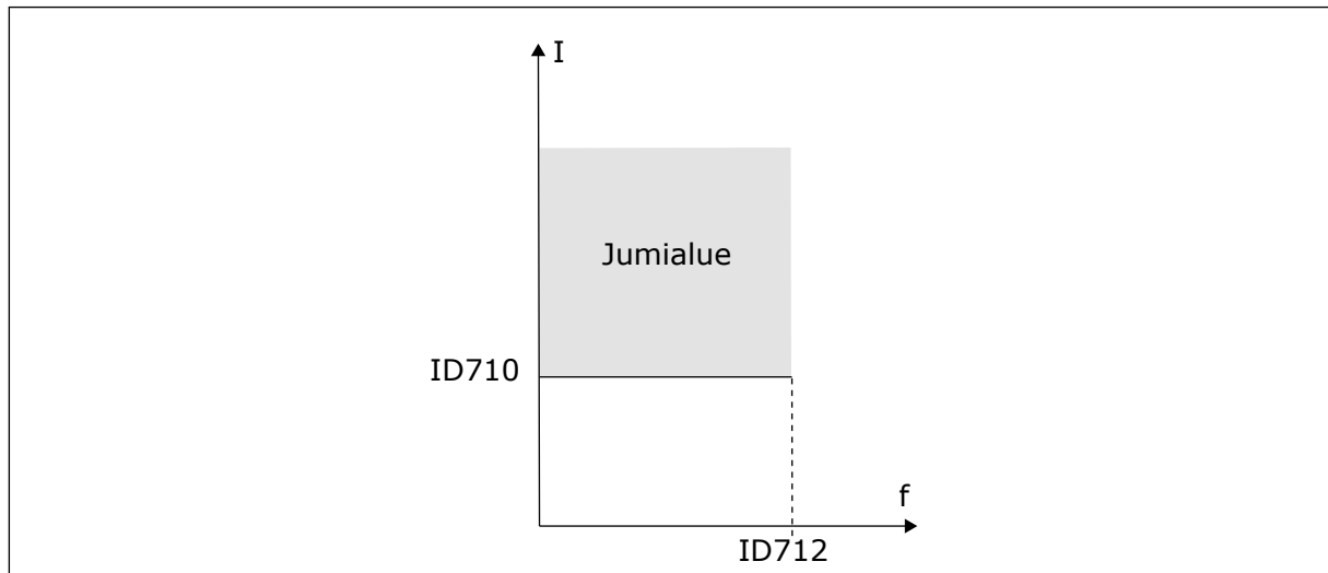
Kuva 58: Jumisuojan asetukset
