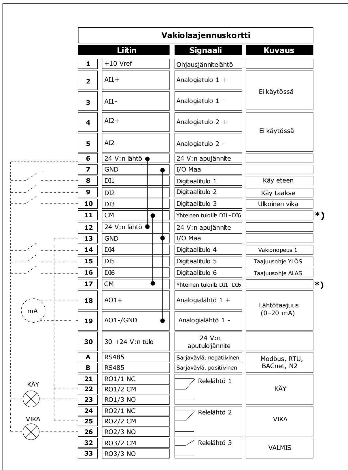
Kuva 14: Moottoripotentiometri -sovelluksen oletusohjausliitännät
