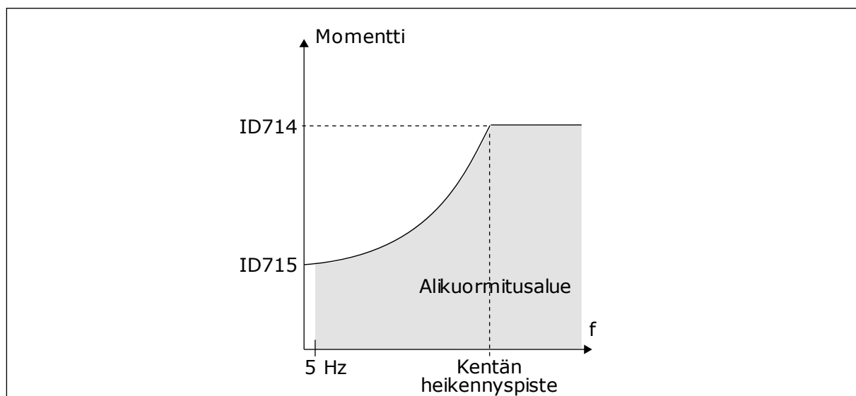
Kuva 59: Minimikuormituksen asetus
