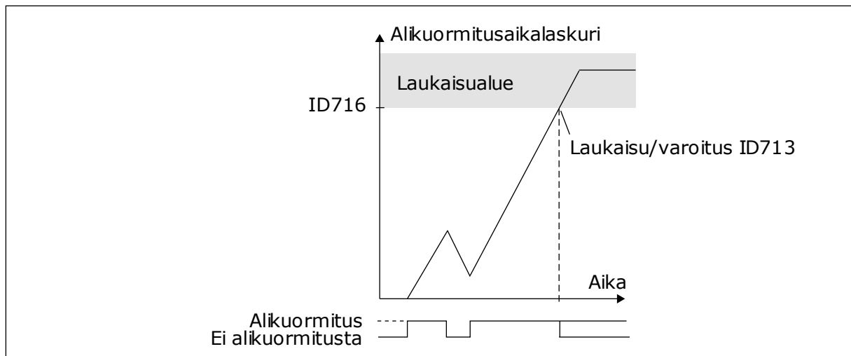
Kuva 60: Alukuormitusaikalaskurin toiminta
