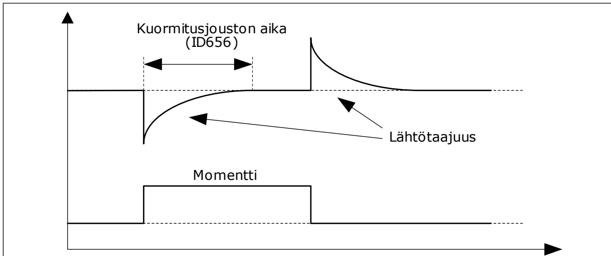
Kuva 21: Kuormitusjoustotoiminto
