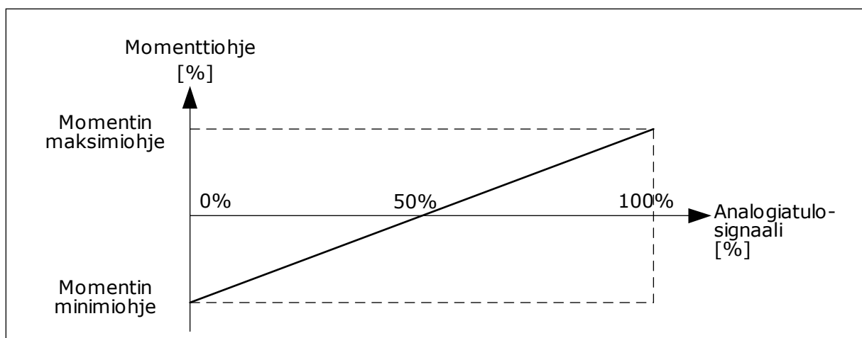
Kuva 34: Momenttiohjesignaalin skaalaus.
