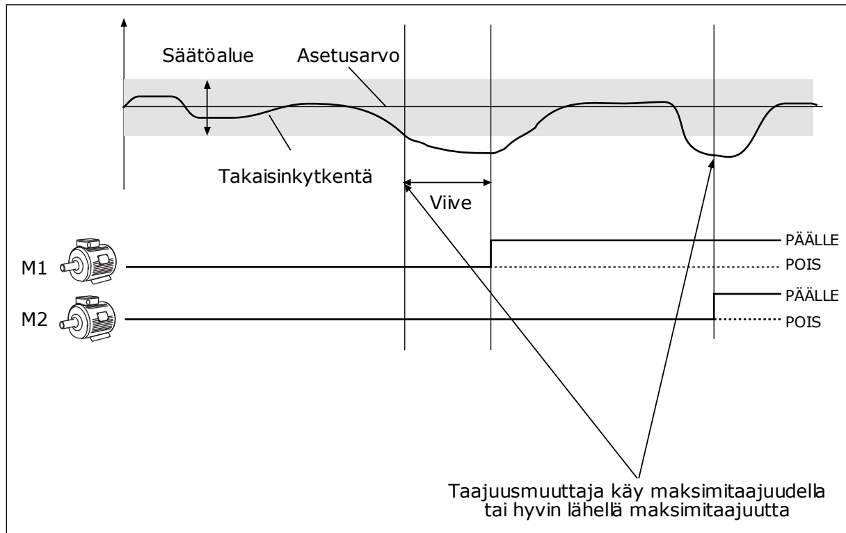
Kuva 79: Monipumpputoiminto
