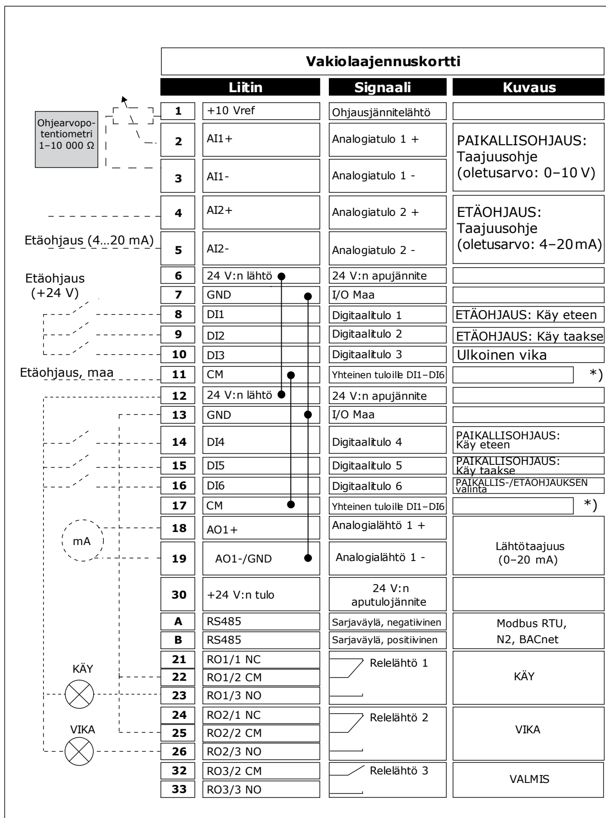
Kuva 6: Paikallis-/etäohjaussovelluksen oletusohjausliitännät
