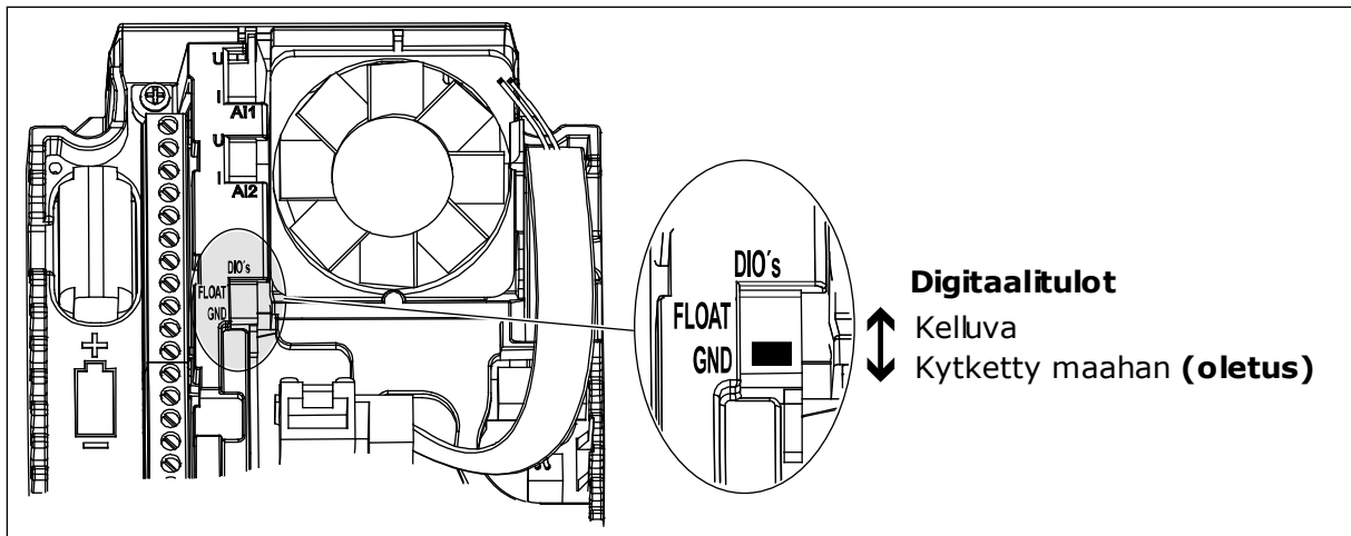
Kuva 7: DIP-kytkin
