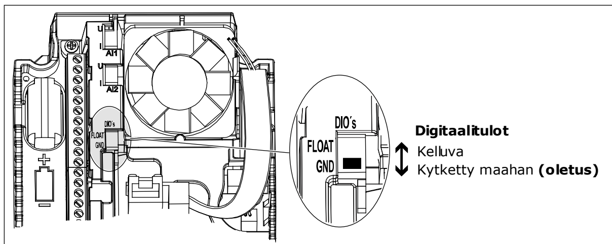
Kuva 11: DIP-kytkin
