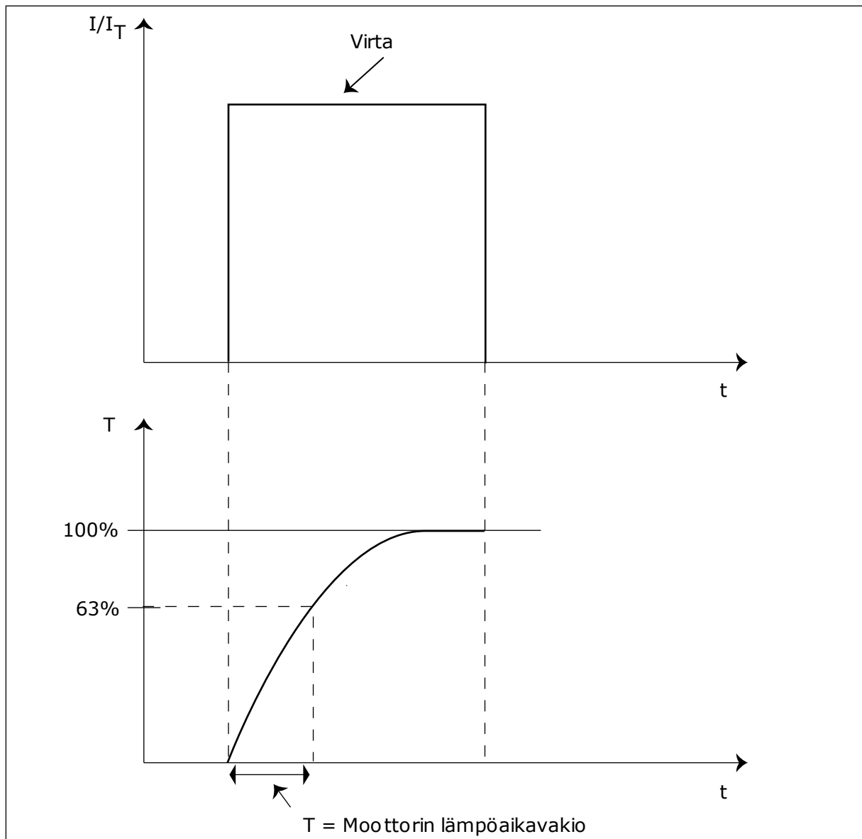
Kuva 56: Moottorin lämpöaikavakio
