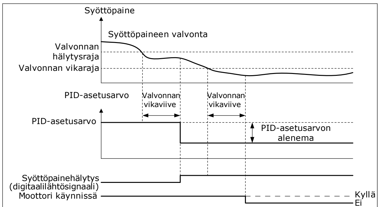
Kuva 78: Syöttöpaineen valvontatoiminto
