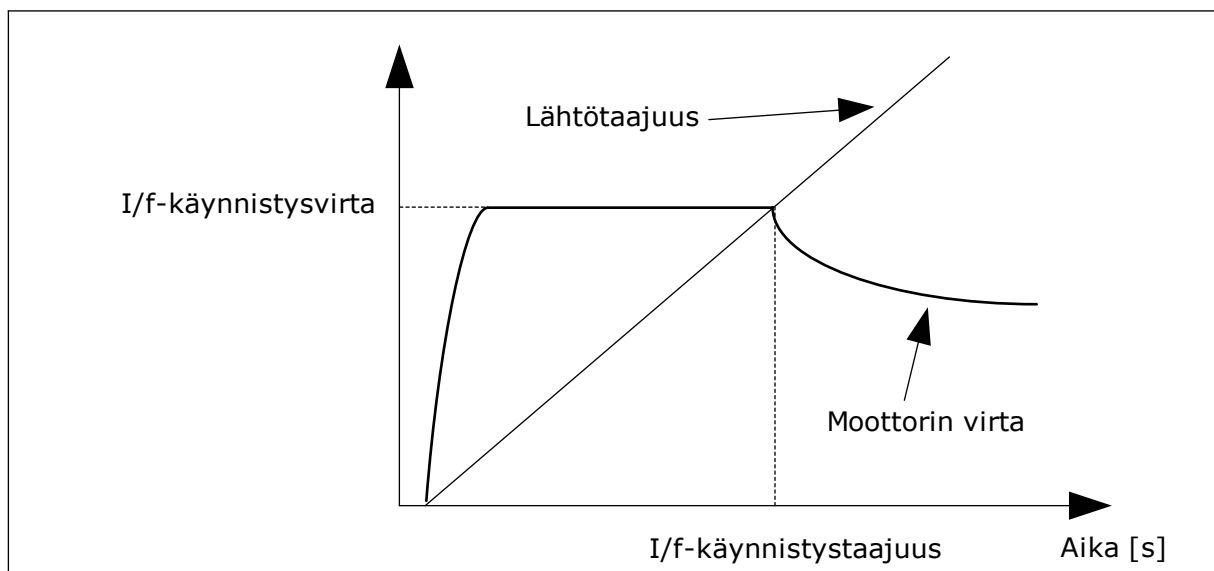
Kuva 25: I/f-käynnistysparametrit
