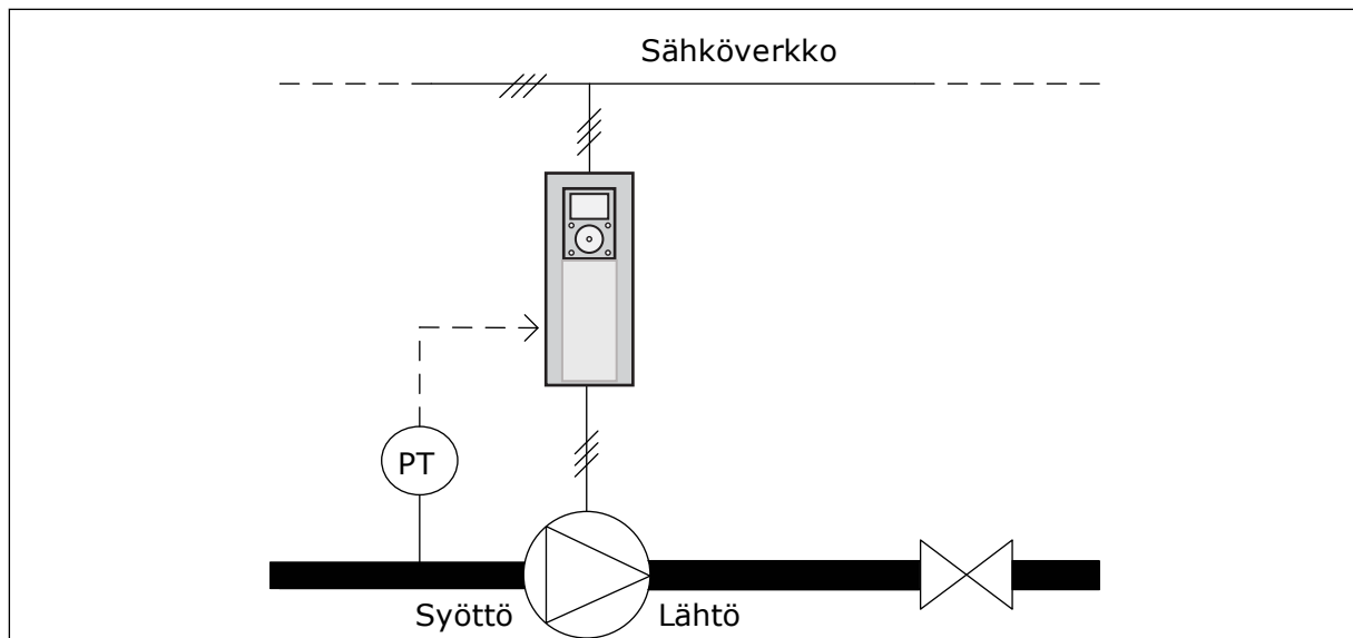
Kuva 77: Paineanturin paikka
