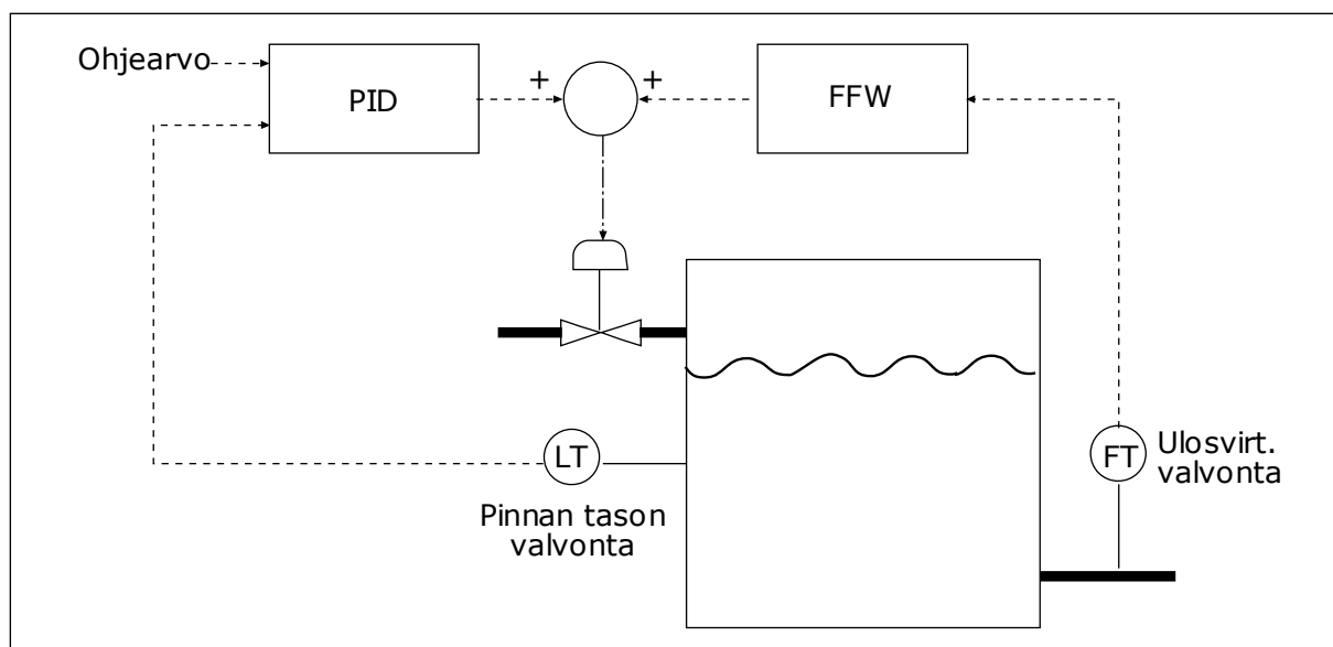
Kuva 70: Myötäkytkentäohjaus.
