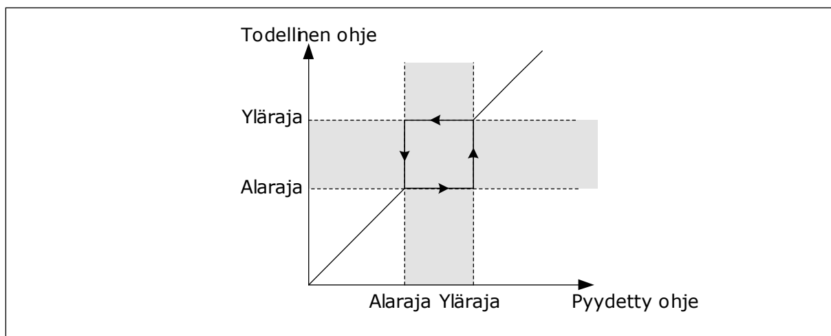
Kuva 53: Estetyt taajuudet
